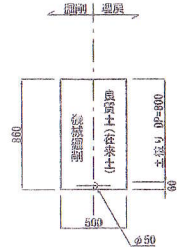
B管土工図 S = 1:20
