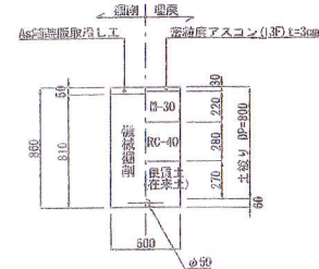
A管土工図 S = 1:20
